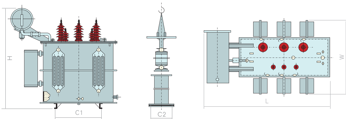
S9-800~31500/35变压器
